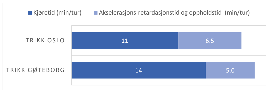
Figur 8.2: Fordelingen av holdeplassetid og reisetid for trikken i Oslo og Gøteborg.
