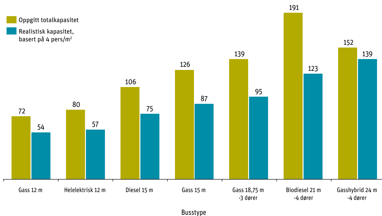
Figur 52: Godkjent totalkapasitet for ulike busstyper, og realistisk kapasitet basert på 4 stående passasjerer per m 2
